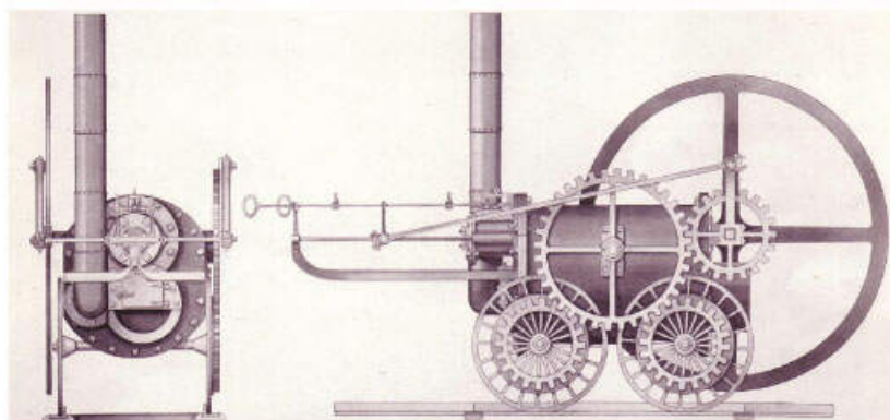
Figura 1.19 La máquina de vapor, emblema de la Revolución Industrial. Locomotora de la compañía Coalbrookdale (1803).
